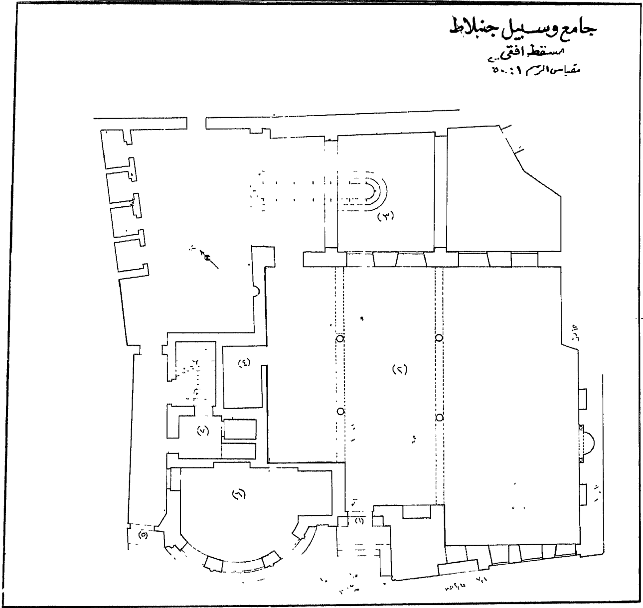
شكل (١١) يبين مسقط أفقي لمدرسة ابن قرقماس المعروفة بمدرسة جنبلات
